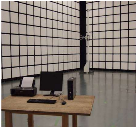
図1 電波暗室
