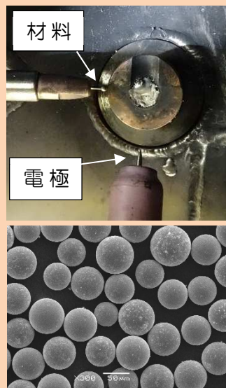
粉末製造装置と製造した粉末
