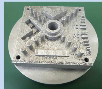
金属積層造形装置と造形品
