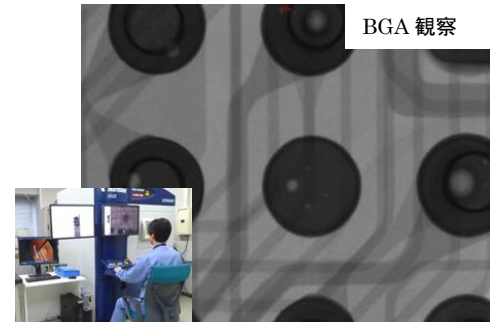
試験番号 13 X線非破壊検査
