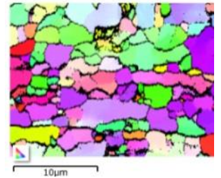
試験番号 7 材料の結晶方位解析
